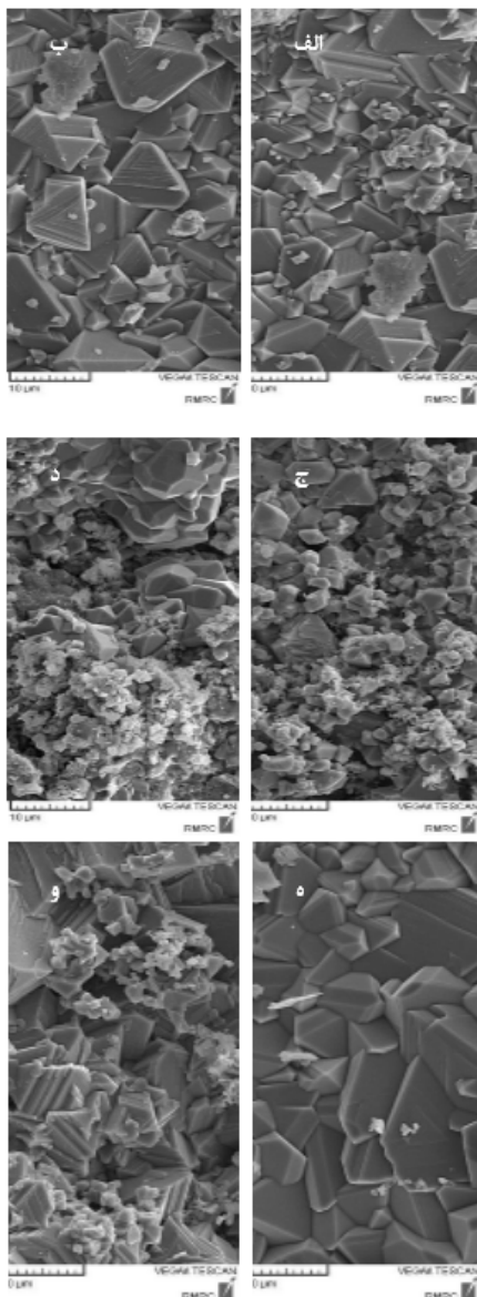
شکل ۵: تصاویر SEM از سطح اکسید شده پوشش‌ها الف و ب) NiAl (ج و د) NiAl-5TiO 2 ، و و) NiAl-5Cr 2 O 3 . تصاویر سمت راست در دمای ۱۰۰۰ و سمت چپ در ۱۲۰۰ سانتی‌گراد
