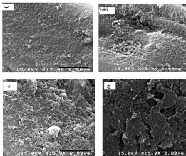
جدول ۱۱: تصاویر SEM حاصل از پارچه ابریشمی پوشش داده شده با محلول ۲۰٪ وزنی اسیدسیتریک و ۱۳٪ وزنی سدیم هاپو فسفیت در دمای جوش با درصدهای MWCNT-COOH (الف) ۴٪ وزنی قبل از شستشو، (ب) ۴٪ وزنی بعد از شستشو، (ج) ۷٪ وزنی قبل از شستشو، (د) ۷٪ وزنی بعد از شستشو
