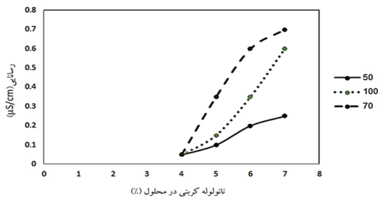
شکل ۴: رسانایی حاصل از پارچه ابریشمی پوشش داده شده با MWCNT-COOH با درصد های ۱٪، ۲٪، ۳٪، ۴٪، ۵٪، ۶٪ و ۷٪ وزنی در دماهای ۵۰ درجه سانتی گراد، ۷۰ درجه سانتی گراد و جوش
