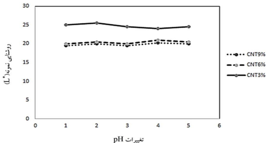
شکل ۵: میزان روشنایی پارچه ابریشمی در حمام حاوی ۳٪، ۶٪ و ۹٪ وزنی نانو لوله کربنی و ابریشم خام در pH های مختلف ۳-۲، ۴-۵، ۶-۷، ۶-۷.
