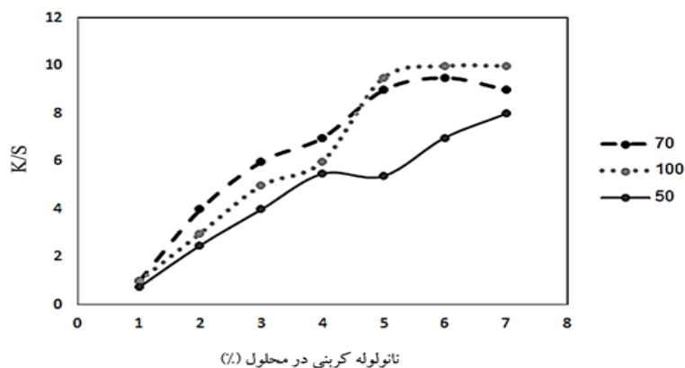
شکل ۳: مقدار K/S در طول موج ۶۰۰ نانومتر، برای پارچه های ابریشمی پوشش داده شده توسط محلول هایی با غلظت ۱٪، ۲٪، ۵٪، ۶٪ و ۷٪ وزنی MWCNT-COOH در سه دمای ۵۰ درجه سانتی گراد، ۷۰ درجه سانتی گراد و جوش
