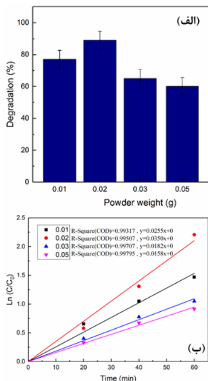
شکل ۱۰: تأثیر مقدار پودر فوتوکاتالیست CoZnAg0.03 در (الف) تخریب و (ب) سینتیک تخریب رنگزای دایرکت یلو
