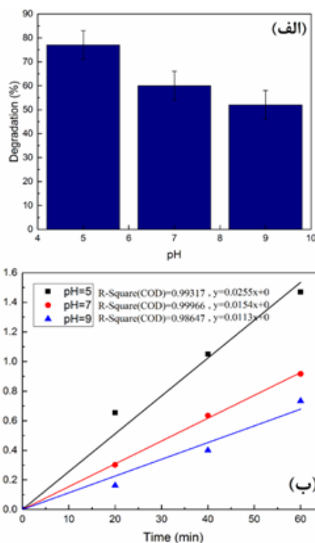
شکل ۹: (الف) درصد تخریب و (ب) سینتیک تخریب رنگزای دایرکت یلو در pH های مختلف در حضور نمونه CoZnAg0.03
