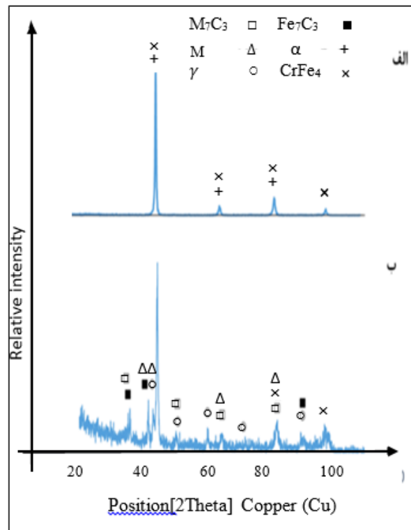
شکل ۴: الگو پراش XRD از سطح روکش با الکتروود E 7018-1 قبل عملیات کربن‌دهی (ب) بعد از عملیات کربن‌دهی.
